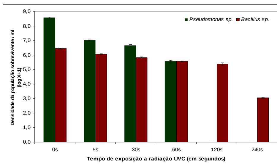
FIGURA 1. Gráfico comparativo das densidades da população sobrevivente à radiação UVC por ml entre representantes dos gêneros Pseudomonas sp e Bacillus sp.
